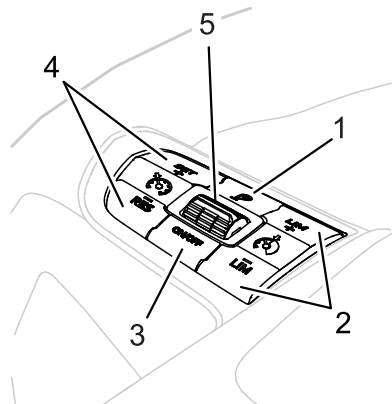
Illustration 34 : Pavé de commande gauche
