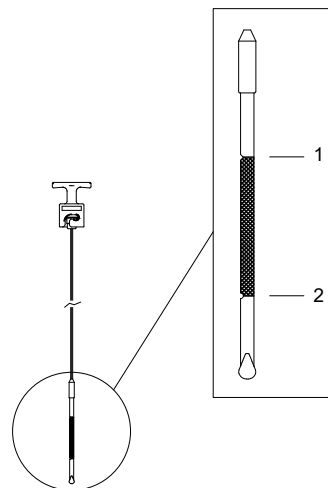
Illustration 57 : Repères de la jauge d'huile à moteur
