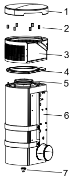
Illustration 59 : Composants du filtre à air du moteur
