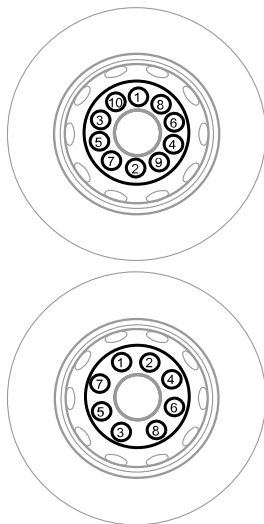
Illustration 62 : Roues à disque centrées par moyeu
