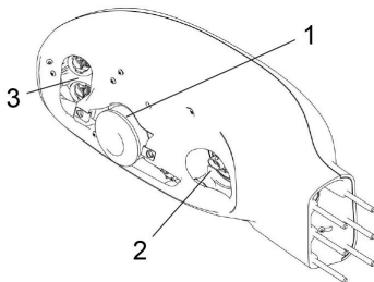
Illustration 60 : Logement de phare — arrière (plaque de protection retirée)
