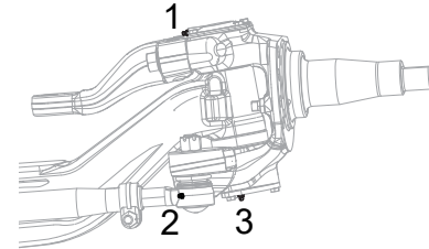
Illustration 54 : Points de graissage pour essieu avant FX-20 PACCAR
