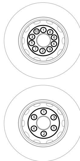
Illustration 63 : Roues à disque centrées par goujons
