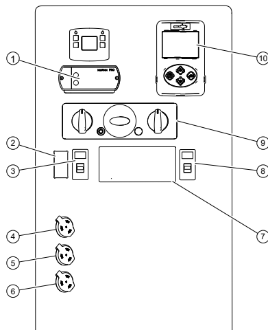
Illustration 24 : Panneau de commande du compartiment couchette
